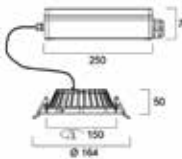
Insaver Slim 150 IP65
